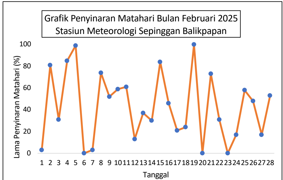
Gambar 2. Grafik Lama Penyinaran Matahari bulan Februari 2025
