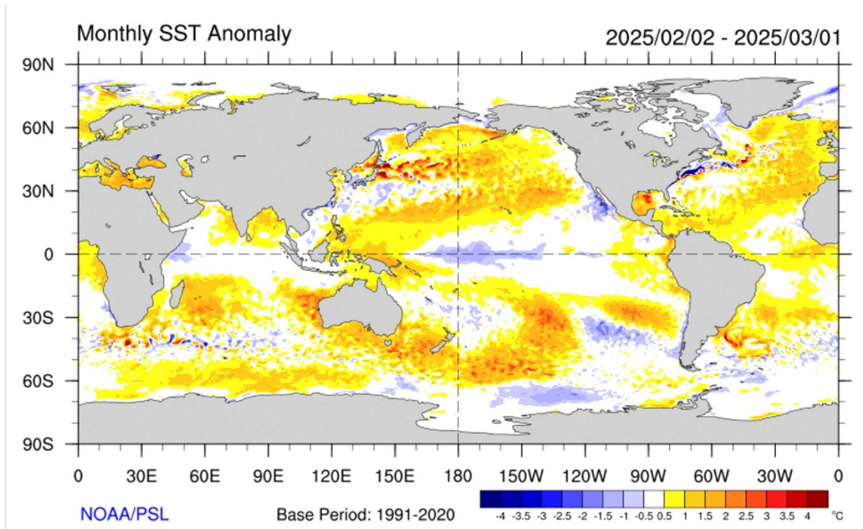
Gambar 11. Peta Anomali SST Februari 2025
