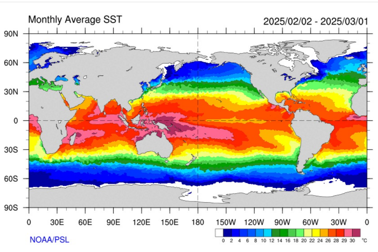
Gambar 10. Peta SST Februari 2025 (Sumber: https://psl.noaa.gov/map/clim/sst.shtml )
