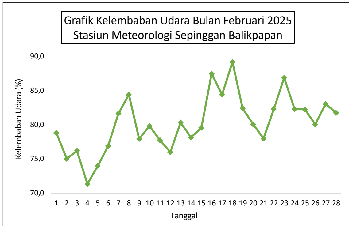
Gambar 4. Grafik Kelembaban Udara bulan Februari 2025
