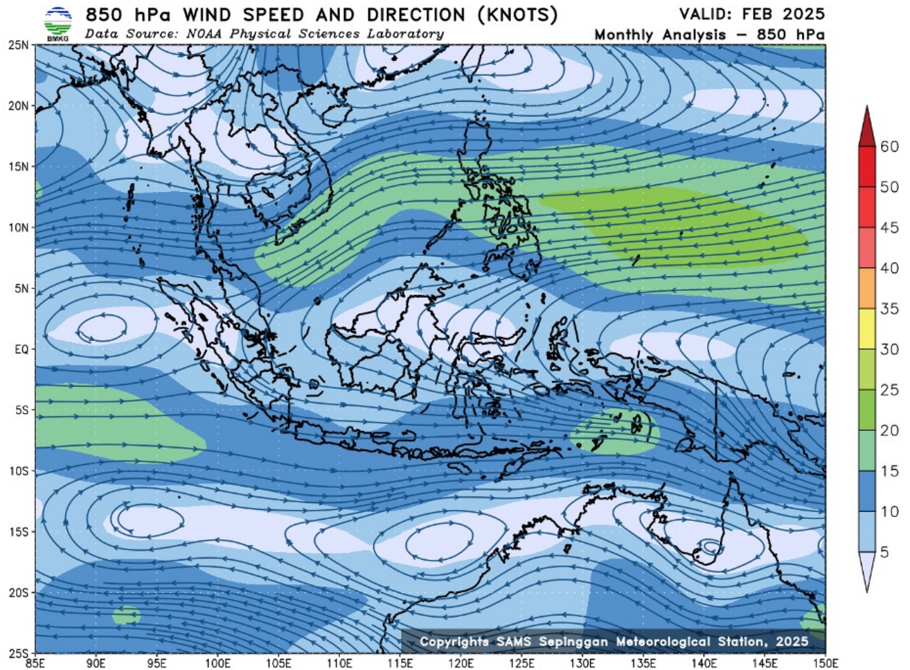
Gambar 6. Rata-rata Bulanan Arah dan Kecepatan Angin 850mb Februari 2025 (Sumber: https://psl.noaa.gov/data/composites/day/ )
