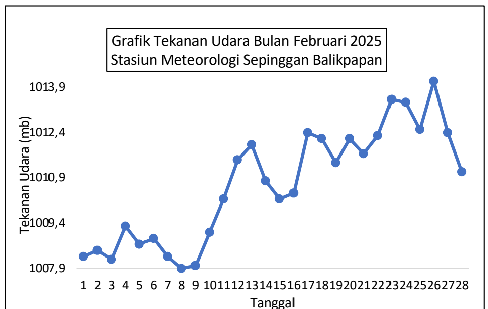
Gambar 3. Grafik Tekanan Udara bulan Februari 2025
