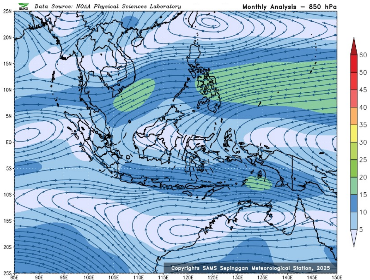
Gambar 7. Rata – Rata Klimatologi Arah dan Kecepatan Angin Bulan Februari (1991-2020)
