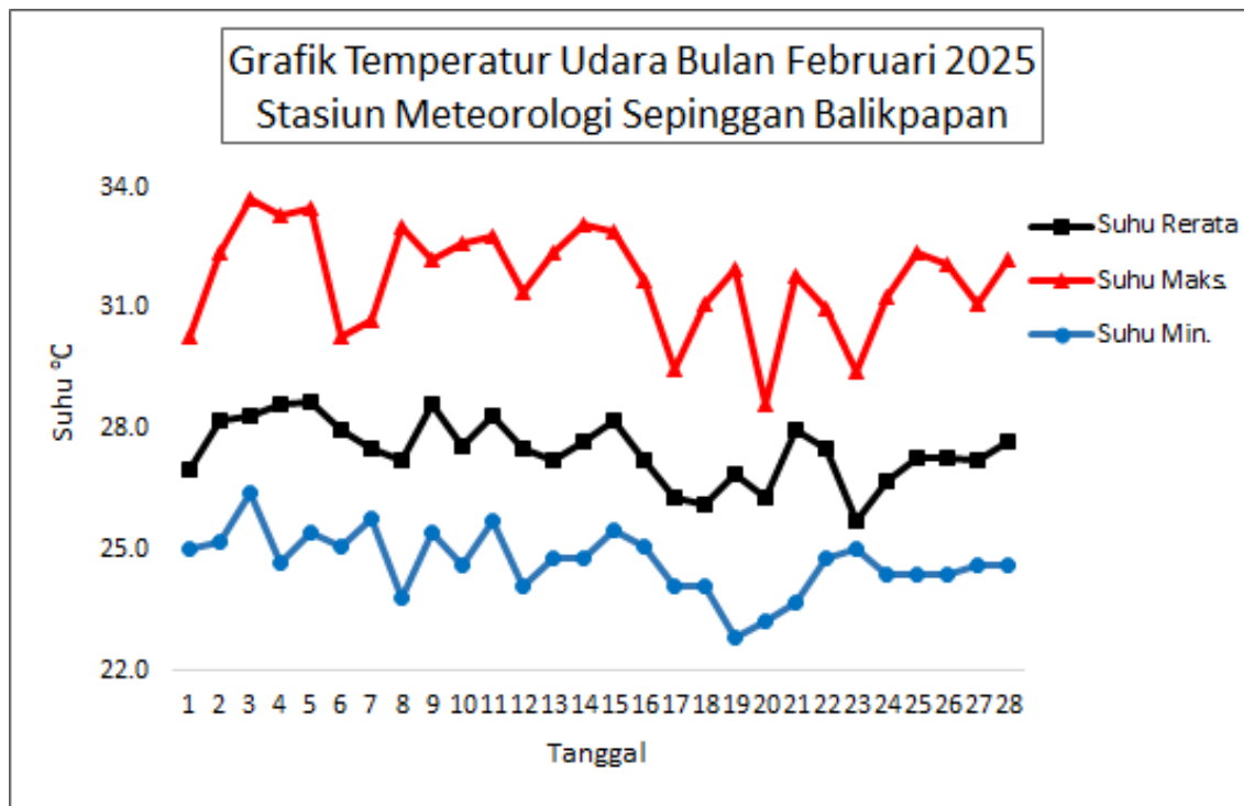
Gambar 1. Grafik Suhu Udara bulan Februari 2025
